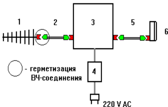
Схема соединений
